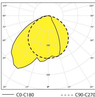
DUNKER65-AS, 2x58W, IP65
