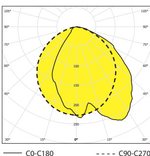
DUNKER65-AS, 4x58W, IP65
