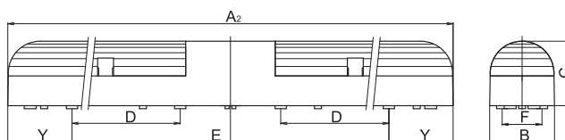
Размеры D и F – шаг крепящих отверстий
